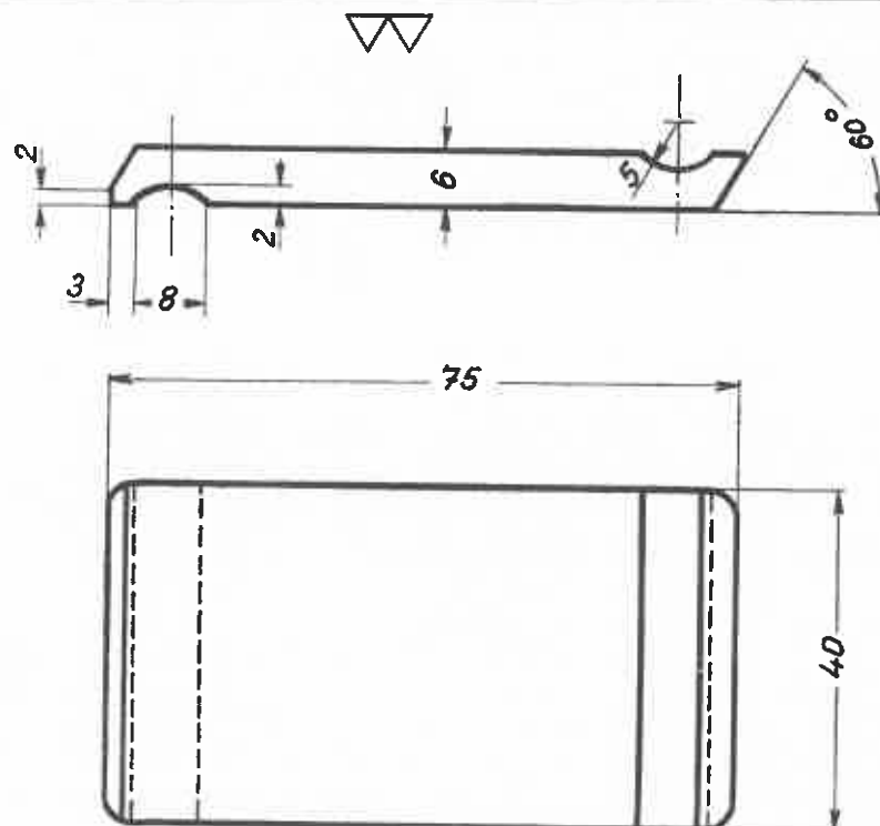
Sperrplatte
