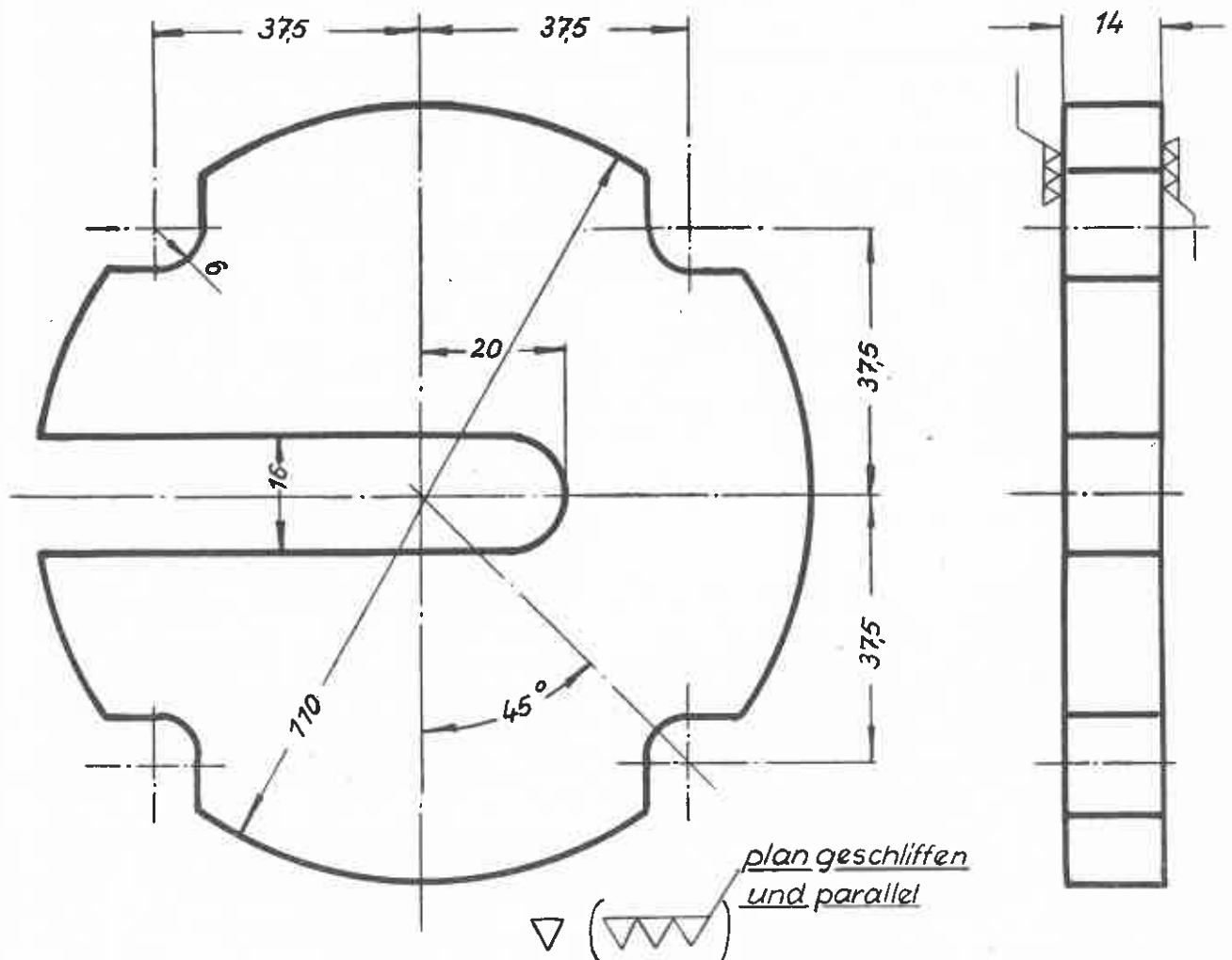
Richtplatte
