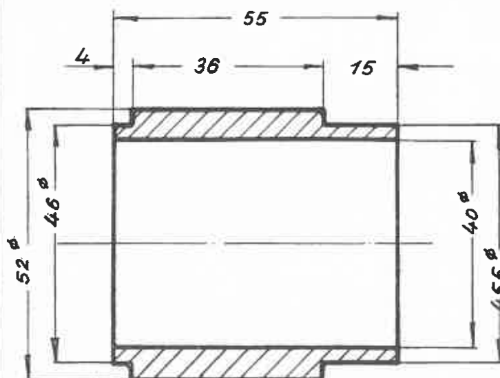
Druckbüchse St. 50.11
