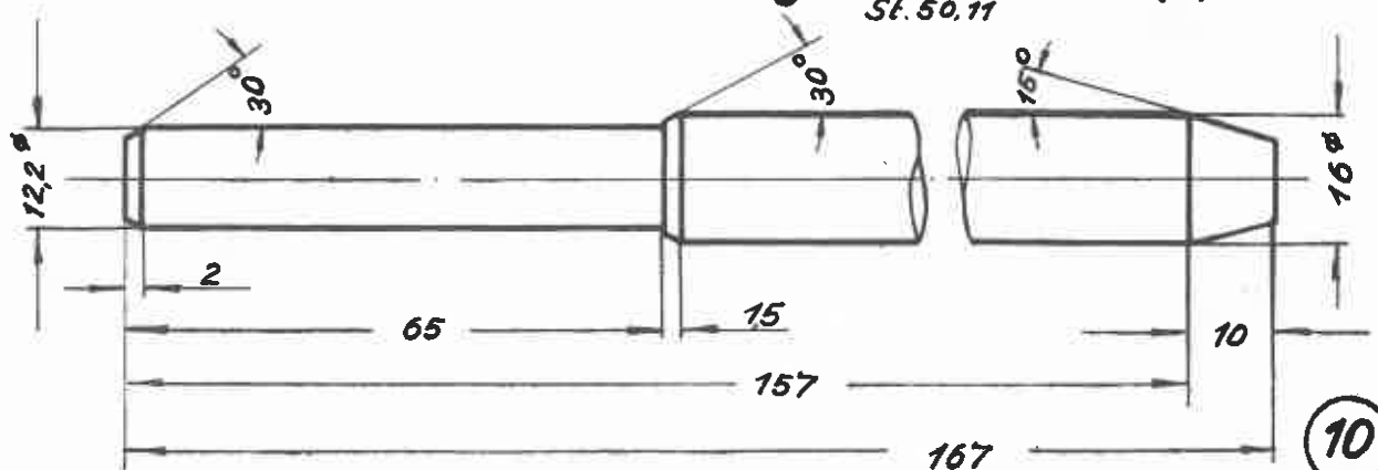
Schlagbolzen
