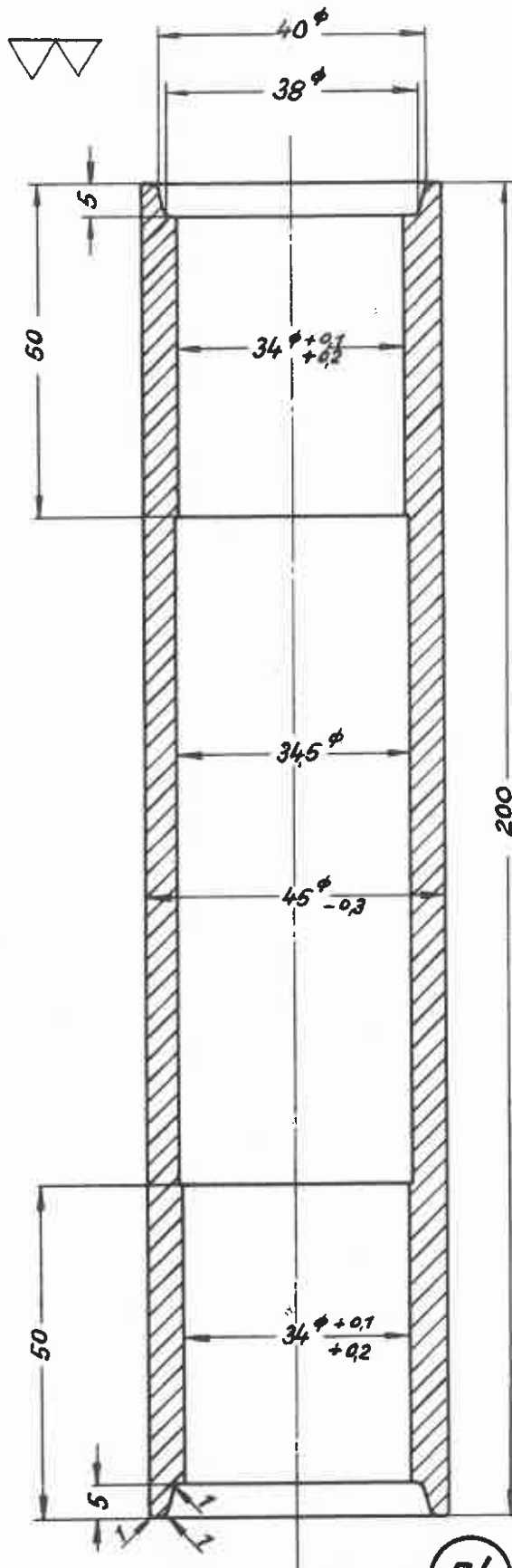
Schlagrohr St. 50.11
