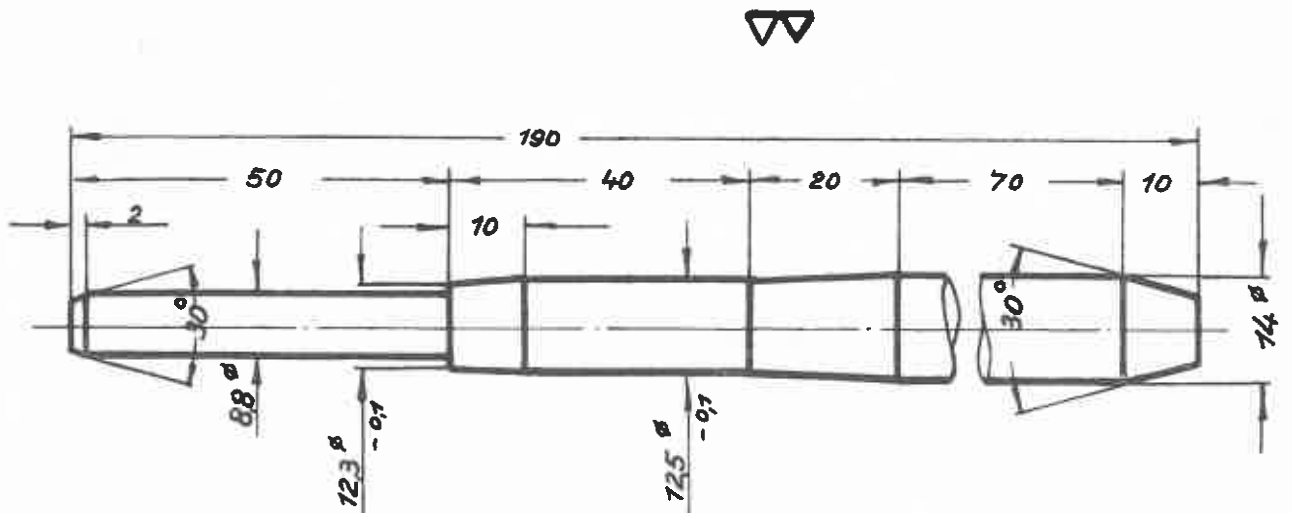
Schlagbolzen St. 50.11
