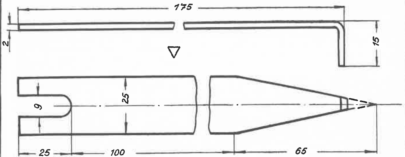
Zeiger Aluminium
