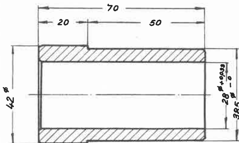
Druckbüchse
