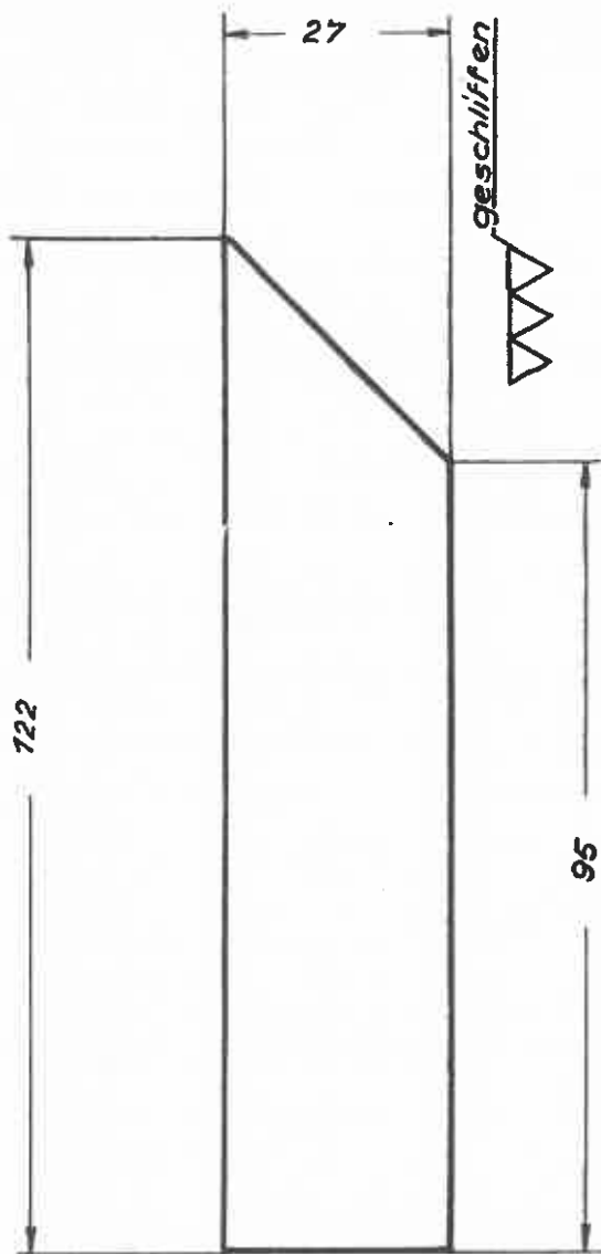
Kontrolleiste St. 50.11
