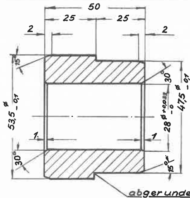
Kontrollbüchse
