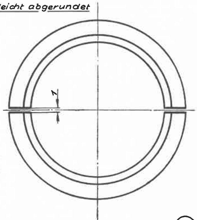
Ringhälften St. 50.11
