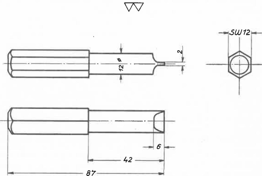
Schraubenzieher-Einsatz
