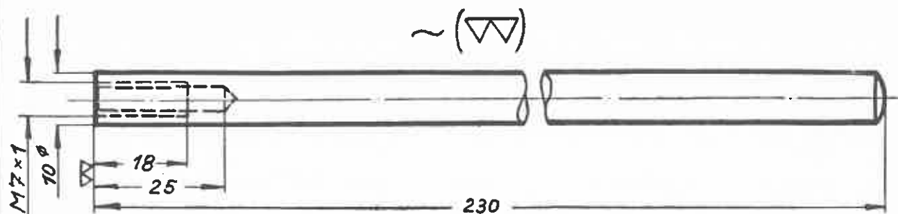
Auszieher St. 50.11
